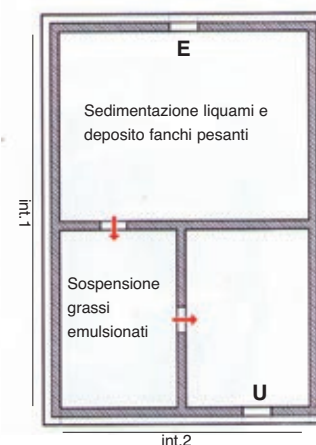
SEZIONE
